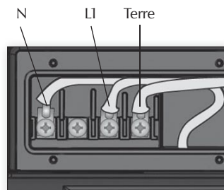
Connexions pour chauffe-eau de 120V (1KW)
