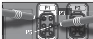
120 VAC au connecteur P1 : P3 et P5
