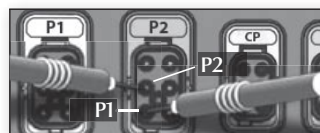
240 VAC au connecteur P2 : P2 et P1
