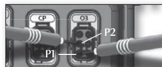
240 VAC au connecteur O3 : P2 et P1
