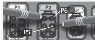
120 VAC au connecteur P2 : P6 et P5
