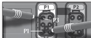
240 VAC au connecteur P1 : P3 et P1
