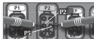
120 VAC au connecteur P2 : P2 et P5
