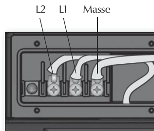
Connexions pour chauffe-eau de 230/240VAC (4KW ou 2 KW)
