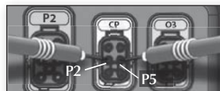
120 VAC au connecteur CP : P2 et P5
