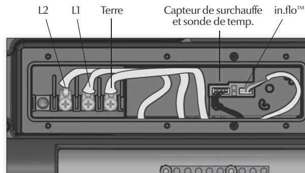
Chauffe-eau 240 VAC (4KW ou 2 KW)
