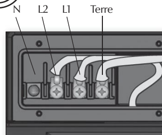
Chauffe-eau 240 VAC (4KW ou 2 KW)
