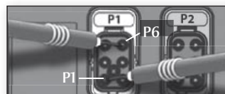
240 VAC au connecteur P1 : P6 et P1
