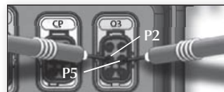
120 VAC au connecteur O3 : P2 et P5
